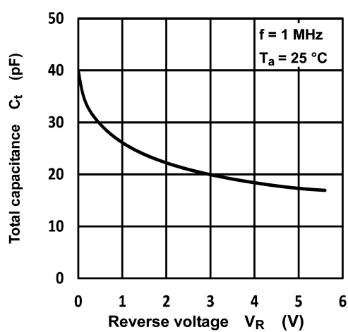
Fig. 7.3 C_t - V_R
