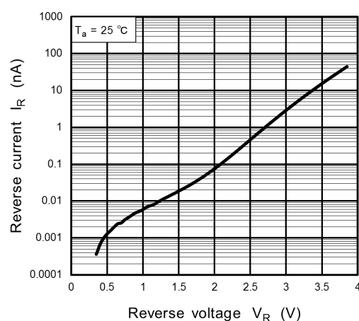
Fig. 7.2 I_R - V_R
