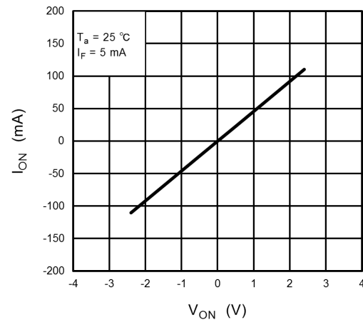
Fig. 12.1.4 I_{ON} - V_{ON}
