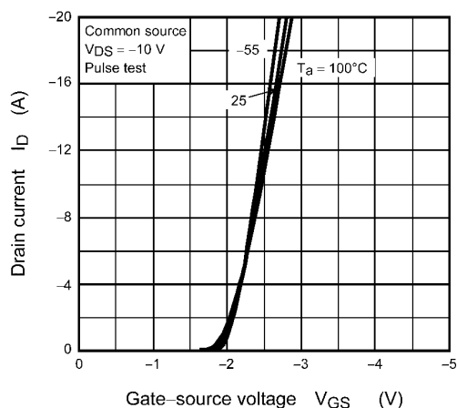
Fig. 8.1.3 I_D - V_{GS}
