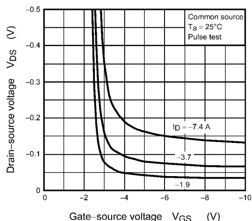
Fig. 8.1.4 V_{DS} - V_{GS}
