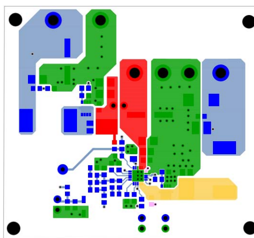
FIGURE 27. TOP LAYER
