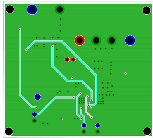
FIGURE 29. 3 rd LAYER
