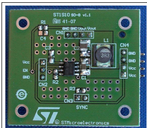
STEVAL-ISA044V1
