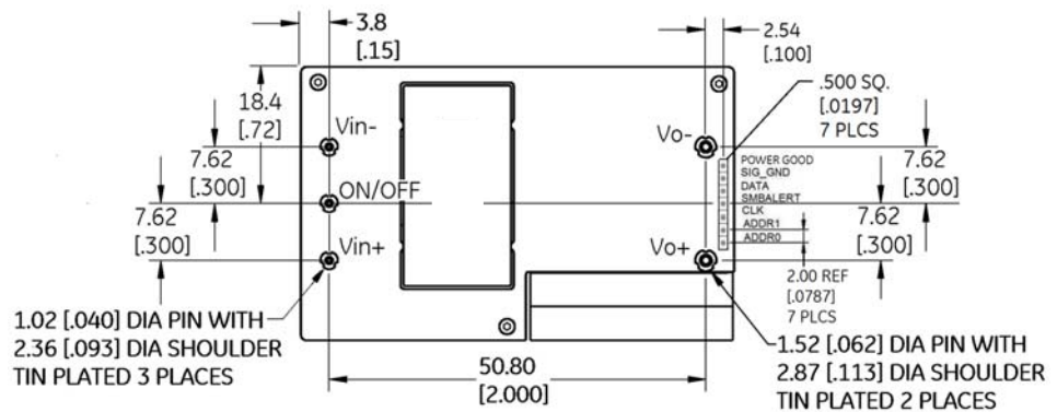
BOTTOM VIEW***
