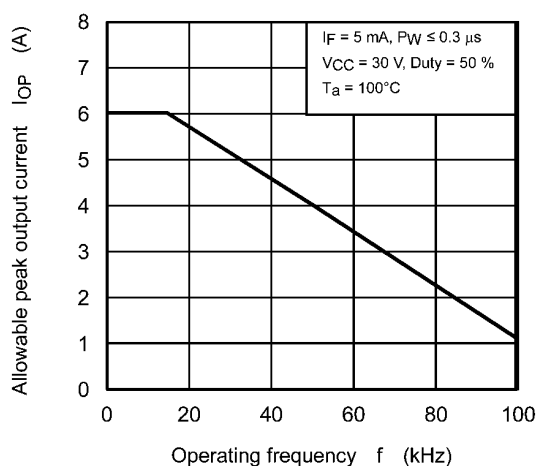
Fig. 12.2.11 I_{OP} - f
