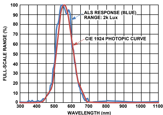
FIGURE 7. ALS SENSITIVITY (Note 14)
