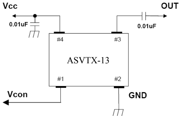
VCTCXO
