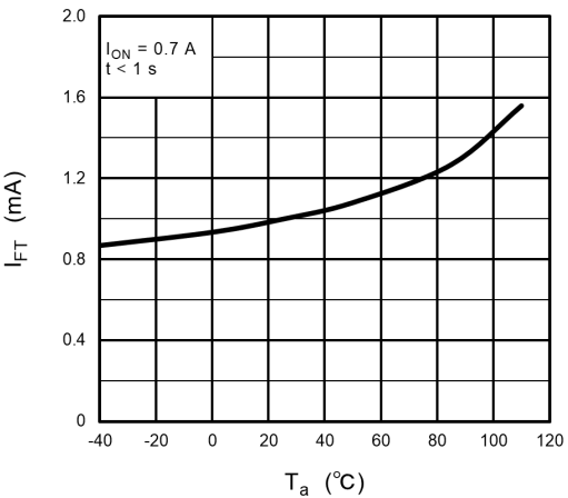
Fig. 14.1.6 I_{FT} - T_a
