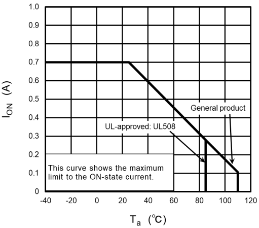
Fig. 14.1.2 I_{ON} - T_a
