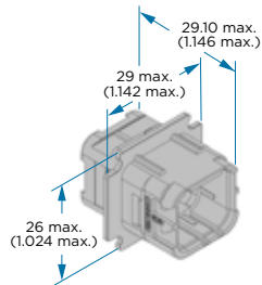
Extender Receptacle
