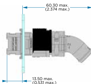
45° Indexable Chimney
