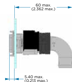
90° Indexable Chimney
