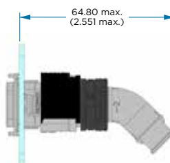
45° Indexable Chimney Tie Wrap
