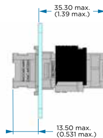
Extender Receptacle
