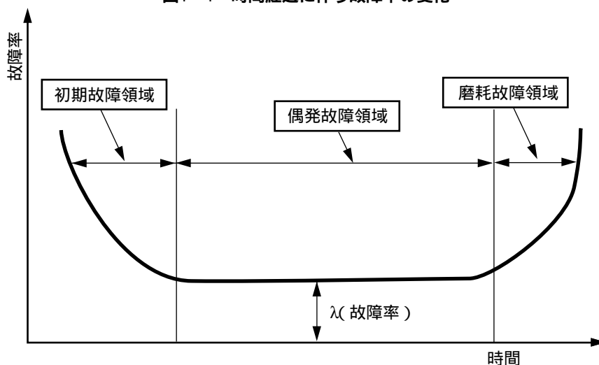
図1-1 時間経過に伴う故障率の変化
